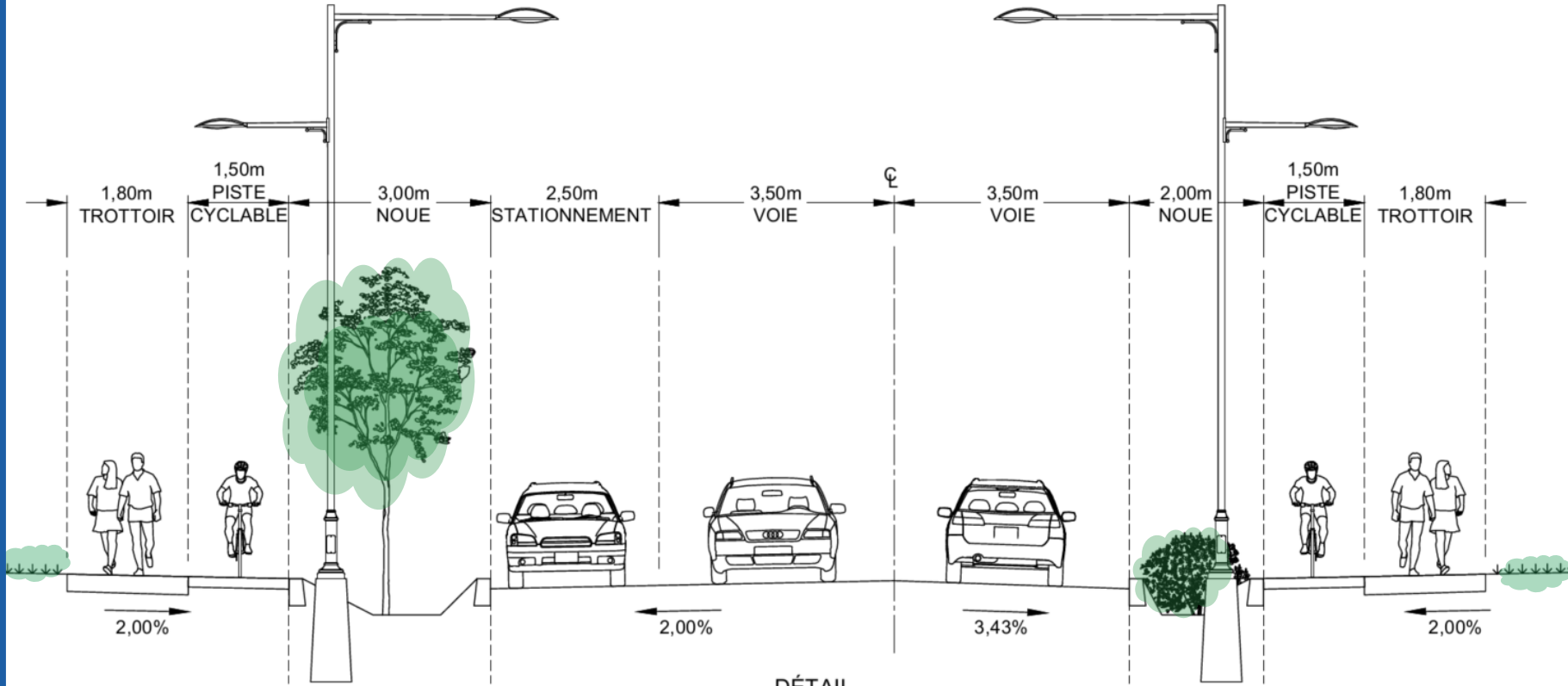
DÉTAIL COUPE DE RUE
